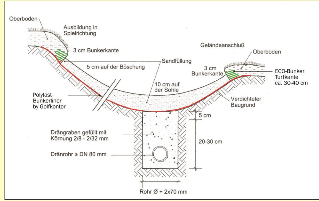
Bunkerschnitt mit Polylast
